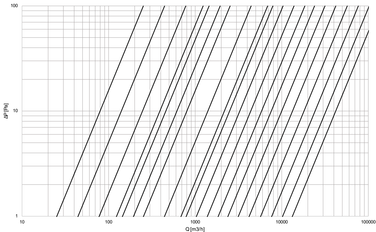
DRUKVAL ASK-1
