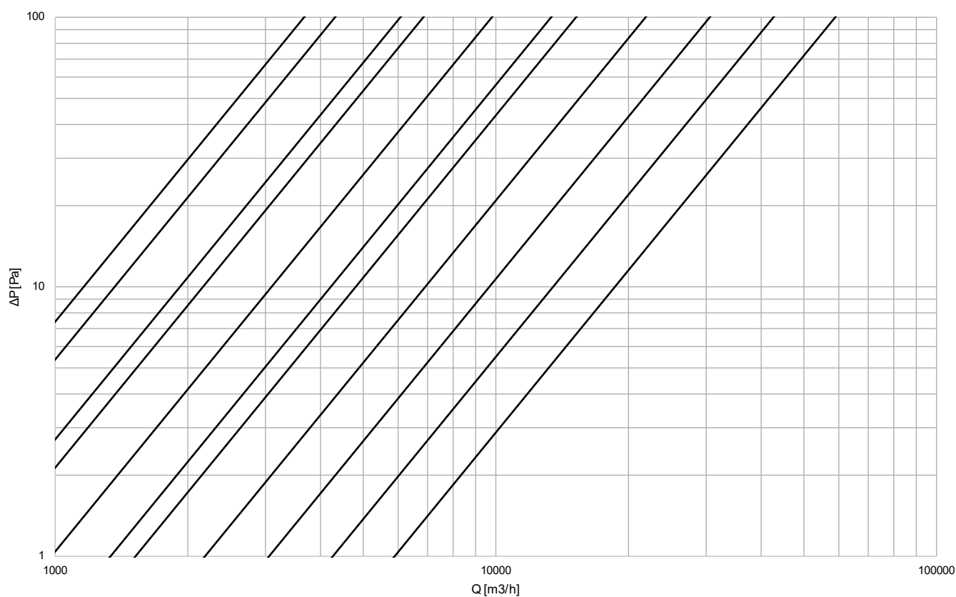
DRUKVAL ASK-2
