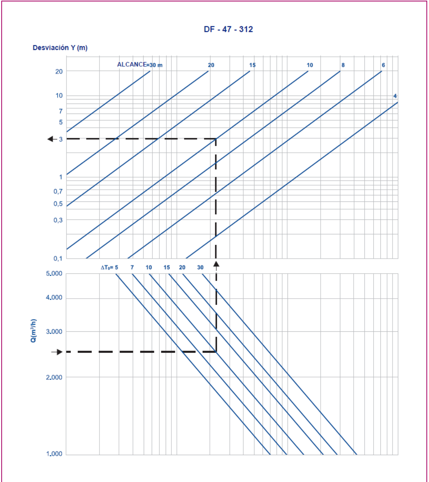
DF-47-3.4.- Desviación vertical de la vena de aire (venas no isotermas).
