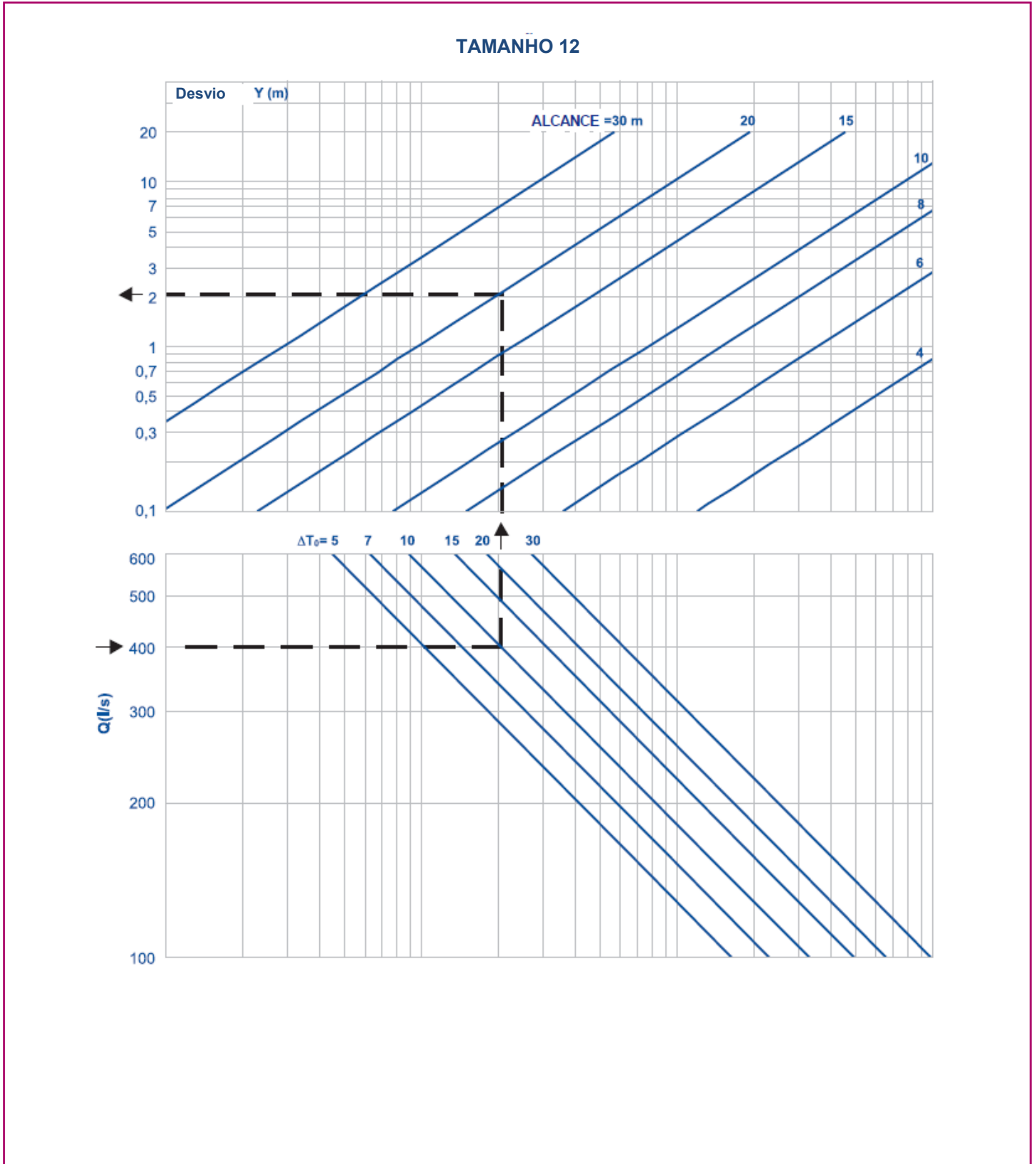
DF-89-3. 3.- Desvio vertical do jacto de ar (jactos não isotérmicos).
