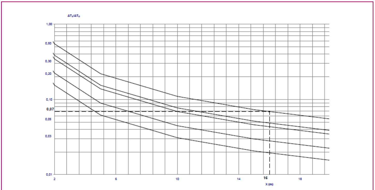
DF-89-5.- Relação entre diferenças de temperatura.
