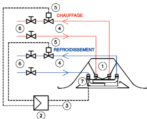
Schéma basique pour installation de débit d'eau variable de 4 tubes.
