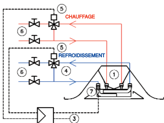
Schéma basique pour installation de débit d'eau constant de 4 tubes.
