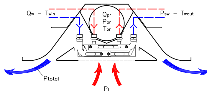
SYSTÈME À 4 TUBES
