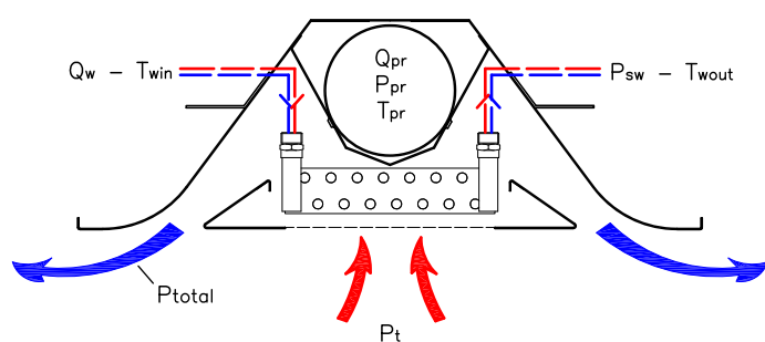
SYSTÈME À 2 TUBES
