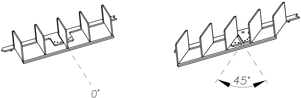
Désign des déflecteurs permettent d'orienter la veine d'air en 4 angles de déflexion (0-15-30-45°)
