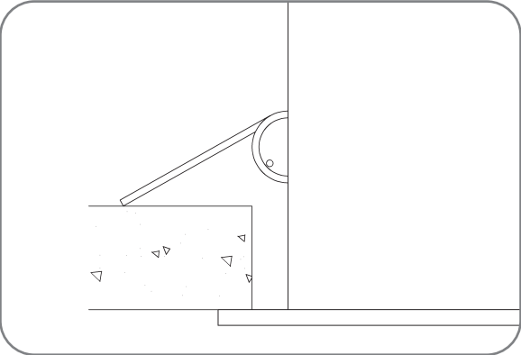
Bevestiging met clips
